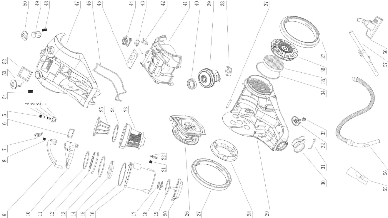
GT-E808爆炸图
